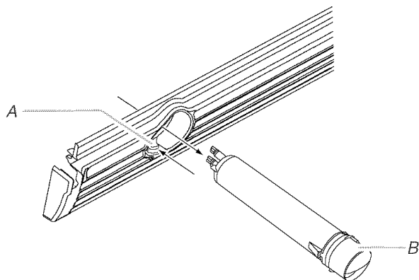
A. Botón eyector B. Tapa
