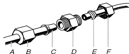
A. Tubería de agua al refrigerador B. Tuerca (provista) C. Bulbo D. Acoplamiento (provisto) E. Férula (adquirida) F. Tuerca (adquirida)
