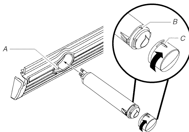
A. Botón eyector B. Ranura en el filtro C. Lomo sobre la tapa
