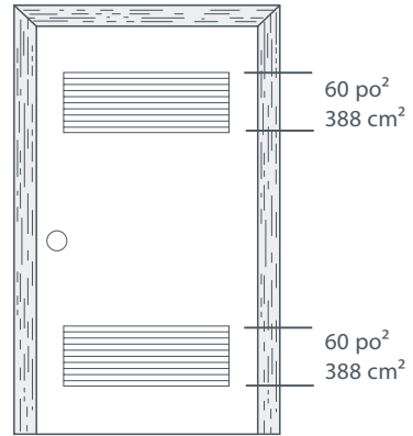
Fig.11 Porte-persienne pour laveuse et sècheuse
