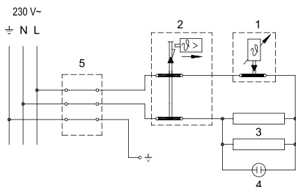
Schema električne vezave
