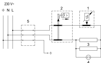
Električna spojna shema
