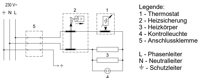
Elektroschaltbild
