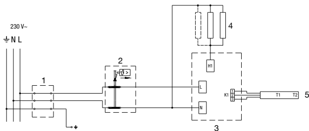
Fig. 6: Skema e lidhjes elektrike
