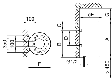
Abb. 1: Senkrechte Montage an die Wand
