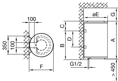
Sl. 1: Uspravno postavljanje na zid
