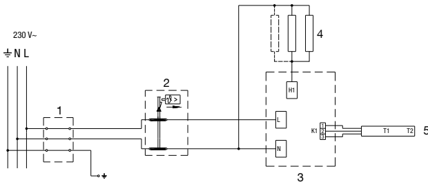
Bild 6: Elektroschaltbild
