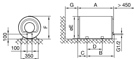
Sl. 2: Ležeča namestitvev na tla
