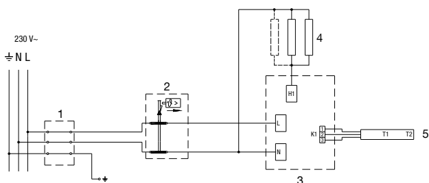
Sl. 6: Shema električne vezave
