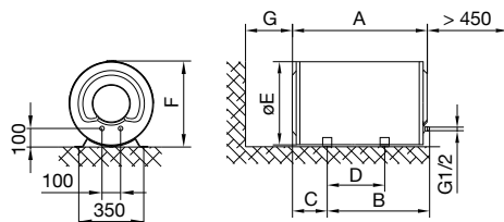
Sl. 2: Ležeće postavljanje na pod
