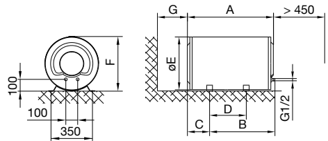
Fig. 2: Montimi horizontal në truall
