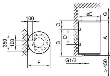
Sl. 1: Vertikalno montiranje na zid
