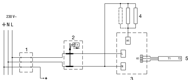
Сл. 6: Шема на електрично поврзување
