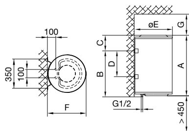
Sl. 1: Pokončna namestitvev na steno
