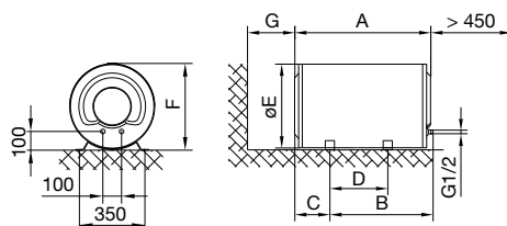
Abb. 2: Waagerechte Montage am Boden
