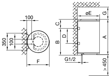
Fig. 1: Montimi vertikal në mur
