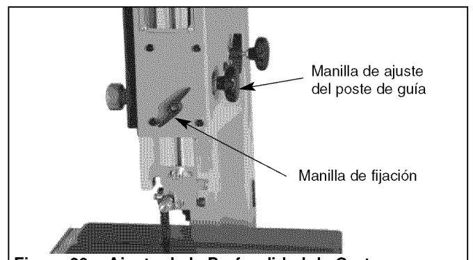
Figura 23 – Ajuste de la Profundidad de Corte
