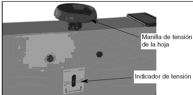
Figura 20 – Ajuste la Tensión de la Hoja
