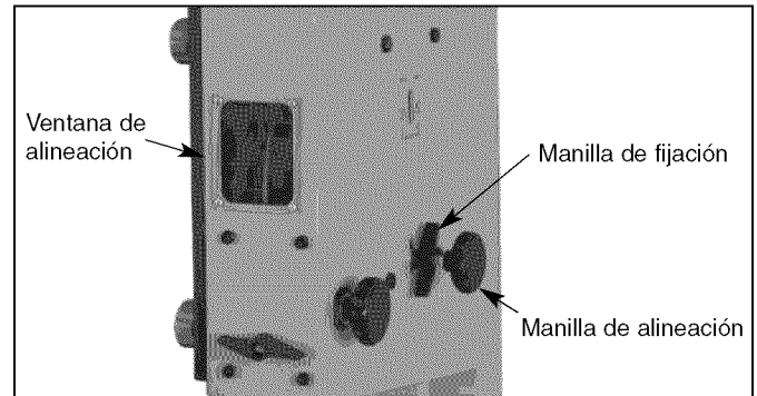
Figura 22 – Alineación de la Hoja de la Sierra
