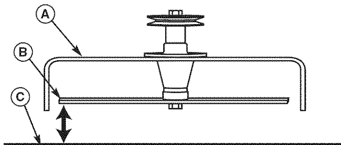
Figura 37. Medir las Puntas del Aspa con el Suelo
