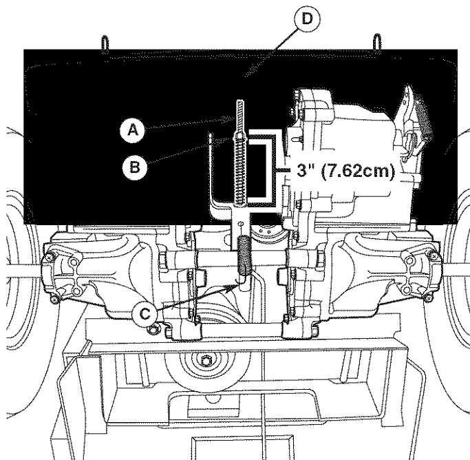
Figura 36. Ajuste del freno A. Varilla del freno B. Tuerca de ajuste C. Resorte de retorno D. Orificio de resorte de retorno
