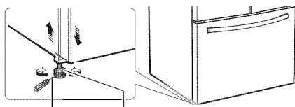
Tournevis à tête plate (-) Molette
