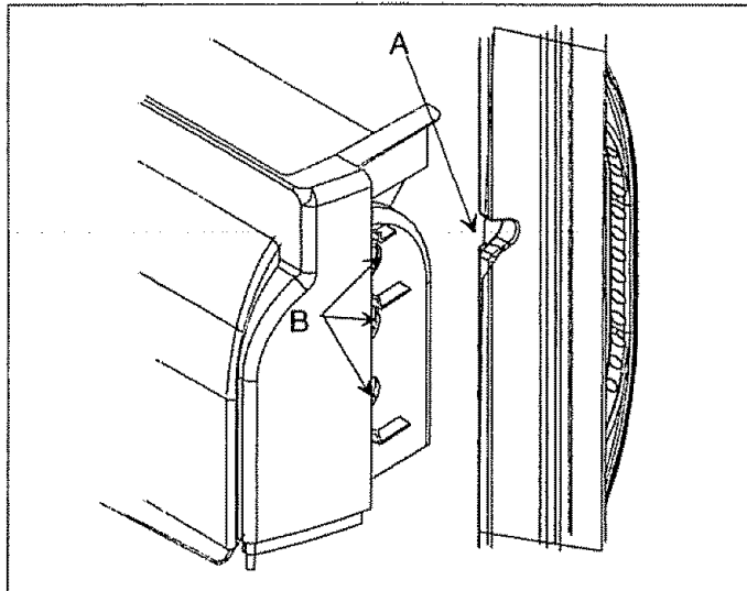
A—Muesca en el pretil de la puerta B—Entradas de aire frío del enfriador para bebidas
