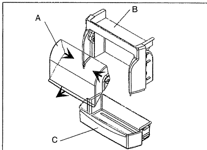
A—Cubierta del enfriador para bebidas B—Base del enfriador para bebidas C—Parte superior del enfriador para bebidas
