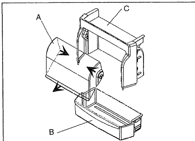
A—Couvercle du refroidisseur de boissons B—Dessous du refroidisseur de boissons C—Dessus du refroidisseur de boissons
