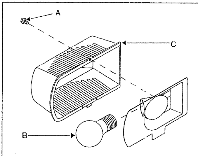
A—Vis B—Ampoule électrique C—Couvre-ampoule
