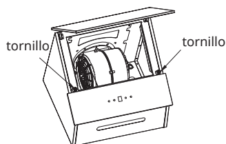
2. Presione hacia abajo el pestillo de plástico y suelte el filtro de la campana. Afloje y retire los dos tornillos del imán fijo.
