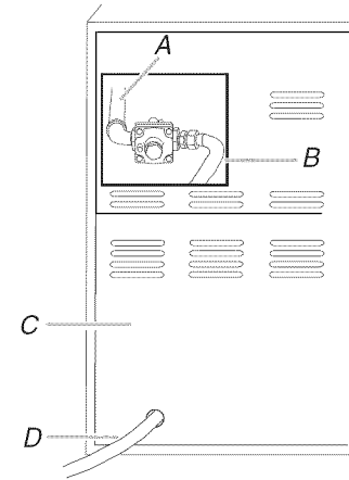
A. Tuyau d'admission de gaz du gril B. Tuyau gris neuf certifié ANSI Z21.54 C. Arrière du gril D. Vers canalisation de propane locale
