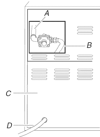
A. Tuyau d'admission de gaz du gril B. Tuyau gris neuf certifié ANSI Z21.54 C. Arrière du gril D. Vers canalisation locale de gaz naturel
