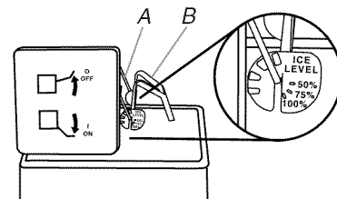
A. Bras de commande en broche B. Bras de réglage du niveau de glace
