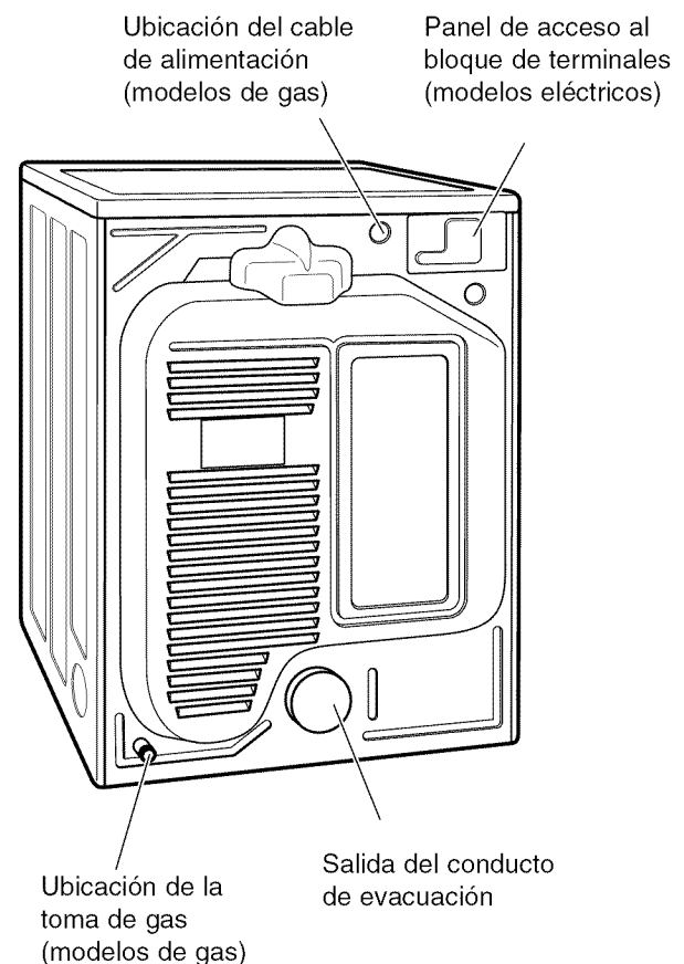
Parte posterior de la secadora
