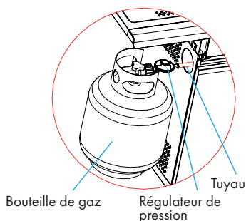
Illustration du raccordement de la bouteille de gaz, du régulateur, du barbecue et du tuyau
